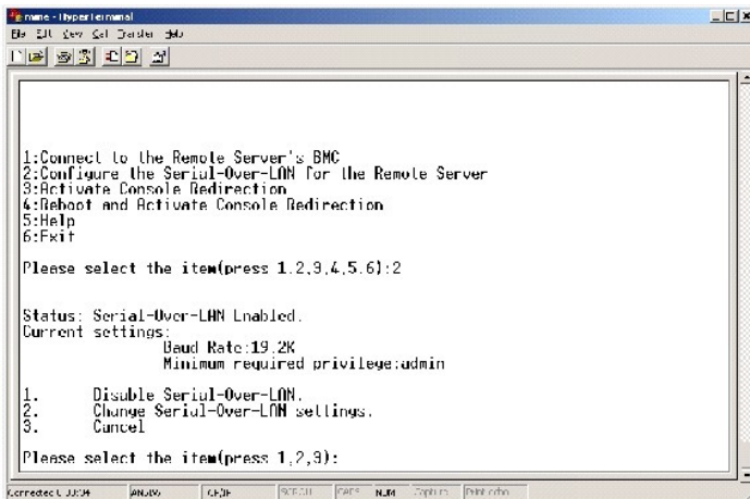
Figura 3-17. Configuración de la comunicación en serie en la LAN para el sistema remoto, ejemplo 1
